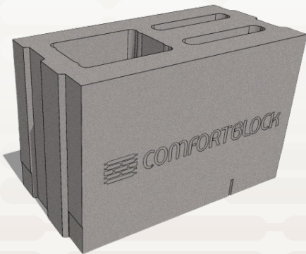
CB-6 Stretcher 6"W x 8"H x 12"L
